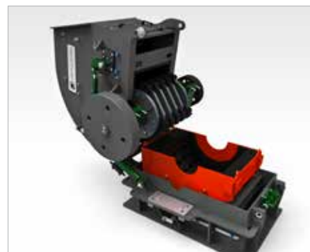
FLEX 1100 MEGA Panizzolo Hammermill Mulino a martelli Panizzolo FLEX 1100 MEGA
